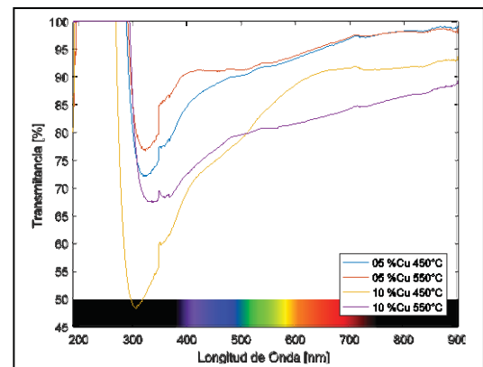
Fig. 3. Espectros de Transmisión UV-Vis para las películas de Al 2 O 3 .
