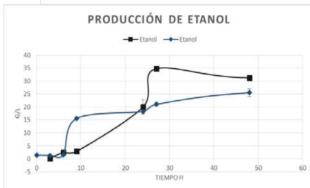
Figs. 4 y 5. Consumo de glucosa y producción de etanol una concentración de sustrato ( S_0 = 60 \text{ g/L} )
