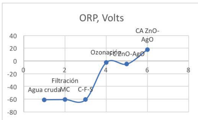
Figura 9. Variación de ORP con ZnO-AgO para fotocatalisis
