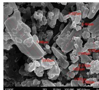
Figura 6. Imagen SEM del polvo de gluconato de zinc producido por la empresa "SAISA".
