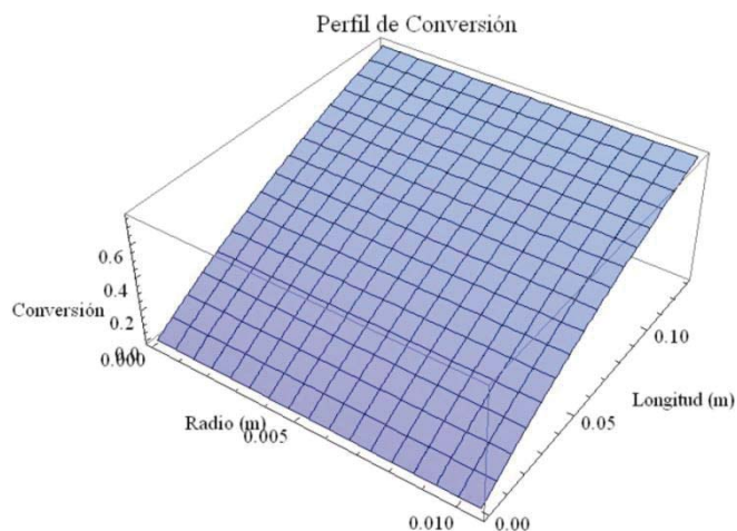
Figura 6. Comportamiento de la conversión de acuerdo al posicionamiento radial y axial en el reactor de lecho empacado
