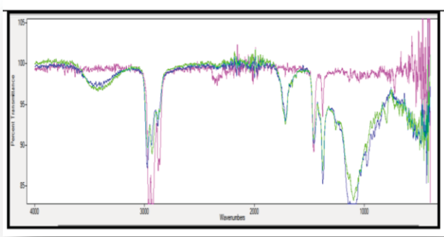
Figura 9. Espectro FT-IR de los lípidos obtenidos. En color verde B. braunii , en azul Scenedesmus sp. el solvente (hexano) en color rosa.
