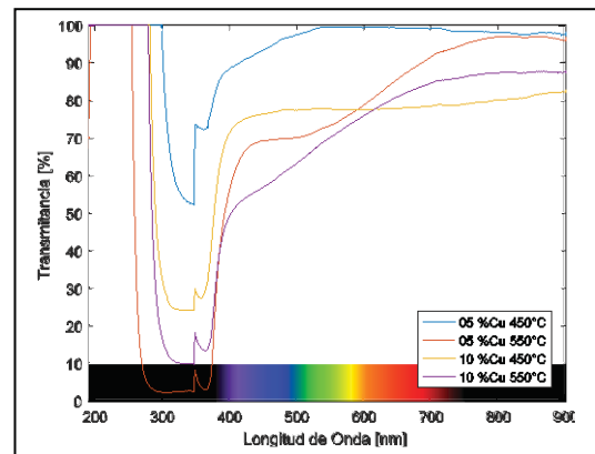
Fig. 2. Espectros de Transmisión UV-Vis para las películas de ZnO.
