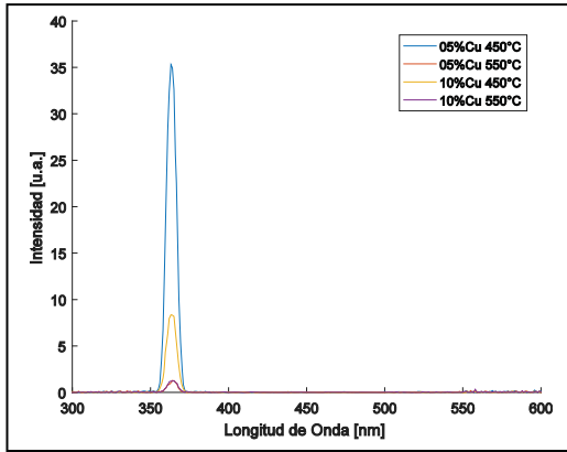
Fig. 8. Espectro de Excitación de las películas de ZnO.
