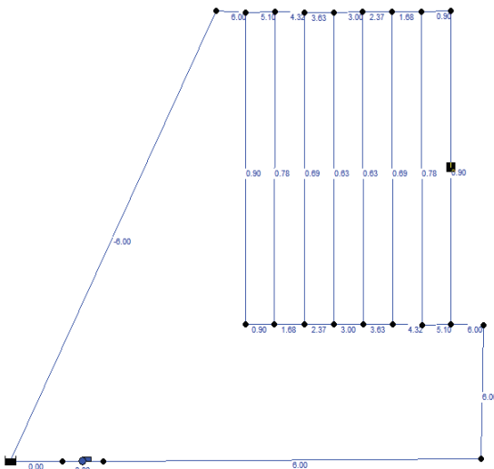
Figura 3. Distribución del flujo con un colector de 8 tubos (cabezal de \frac{3}{4} " y tubos de distribución de \frac{3}{8} ").
