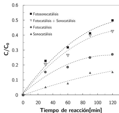
Figura .11.- Cuantificación del efecto sinérgico entre fotocatalisis y sonocatálisis, mineralizados + intermediarios..
