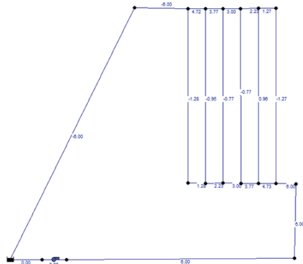
Figura 2. Distribución del flujo en un colector solar de 6 tubos (cabezal de \frac{3}{4} " y tubos de distribución de \frac{1}{2} ").
